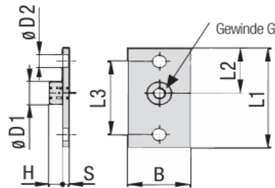
STAUFF Größe 1
